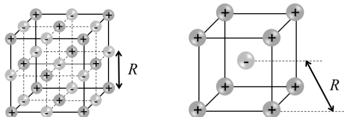
図2 (左) 塩化ナトリウム構造 (右) 塩化セシウム構造
